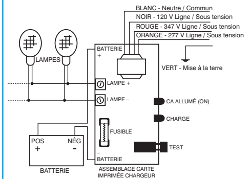
Configuration de la batterie terminal sur la carte de circuit imprimé du chargeur
