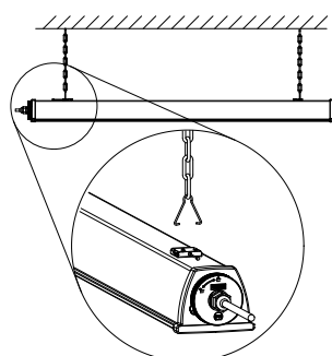
EN SUSPENSION
