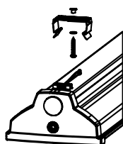
EN SURFACE
