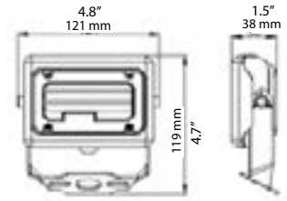
Yoke
