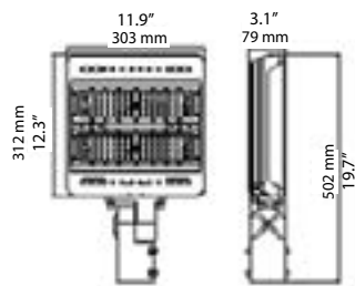
Slipfit*
