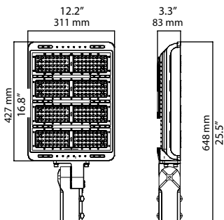
Slipfit*
