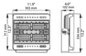
Yoke
